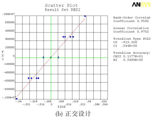
图3 层间变形与地震作用( F_{X1} )样本分布散点图
