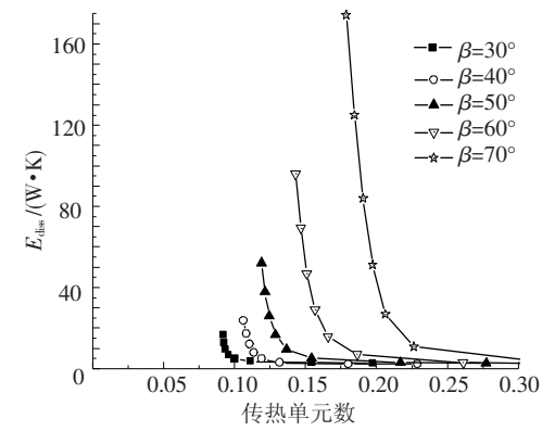
图3 火积耗散率随换热器传热单元数变化曲线
