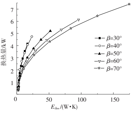
图6 换热量随火积耗散率变化曲线
