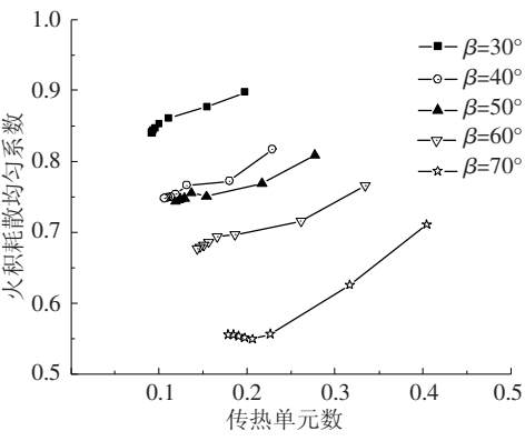
图7 火积耗散均匀性系数随传热单元数变化曲线
