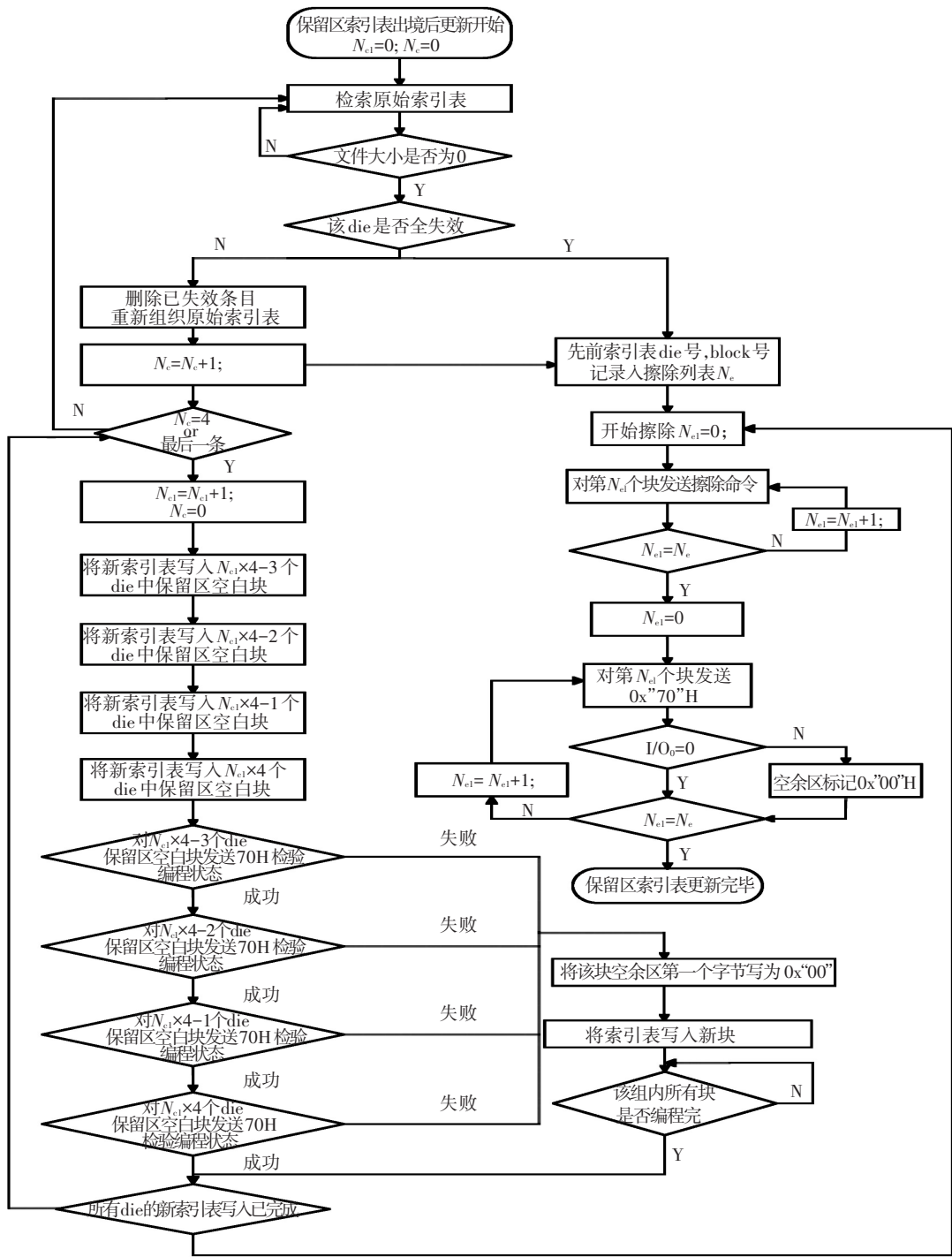
图 1 索引表更新流程
