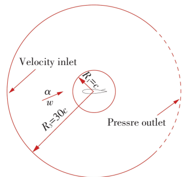
图 3 计算域及边界条件
