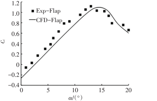
图 7 计算值与实验值对比
