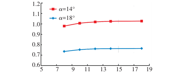
图 5 升力系数随网格数量的变化
