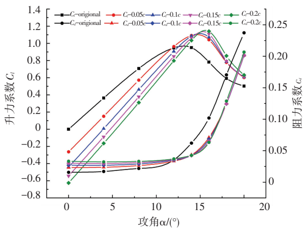
图 11 不同长度翅片翼升阻力系数
