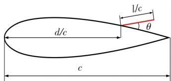
图 2 仿生翅片翼计算模型
