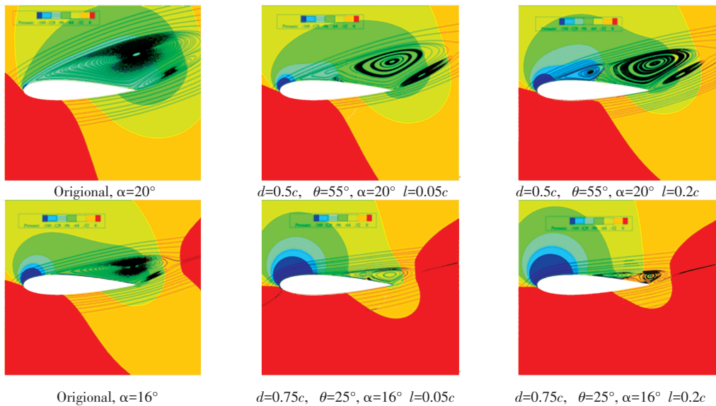
图 13 不同长度翅片翼流场比较
