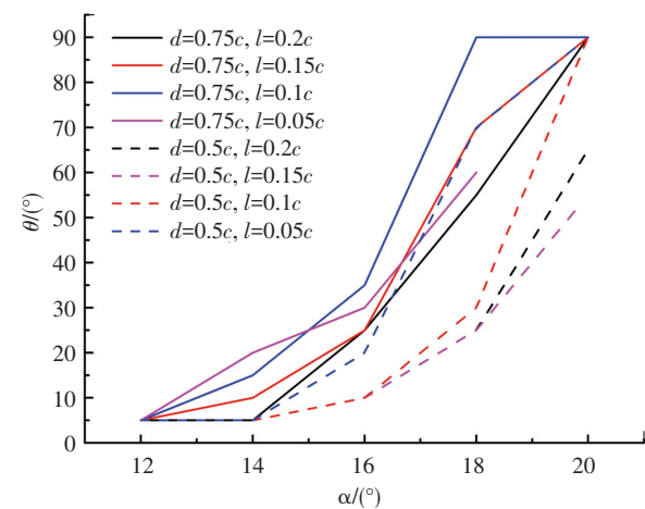
图 15 最佳角度随攻角变化
