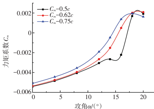
图 9 襟翼力矩系数变化曲线
