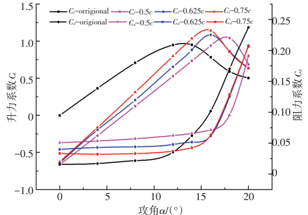
图 8 升阻力系数曲线
