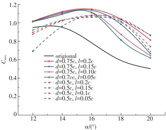
图 14 最大升力系数随攻角变化
