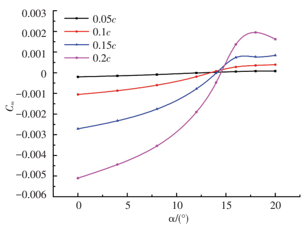
图 12 襟翼力矩系数变化曲线
