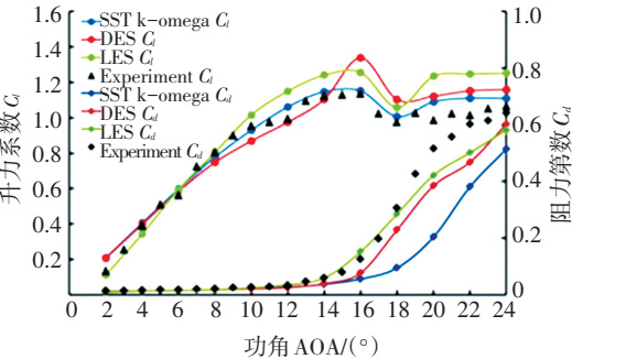
图 6 升阻力系数
