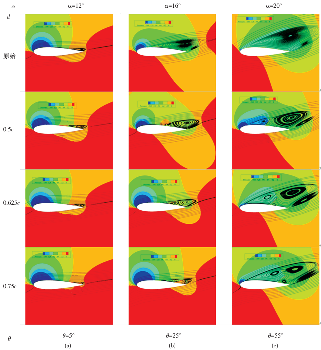
图 10 不同位置处仿生翅片翼的压力云图及流线图 Fig.10 Pressure cloud diagram and streamline diagram of fin wing at different positions
