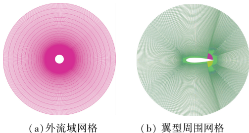
(a) 外流场网格
