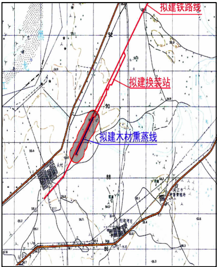
图 7 环境防护距离示意图
