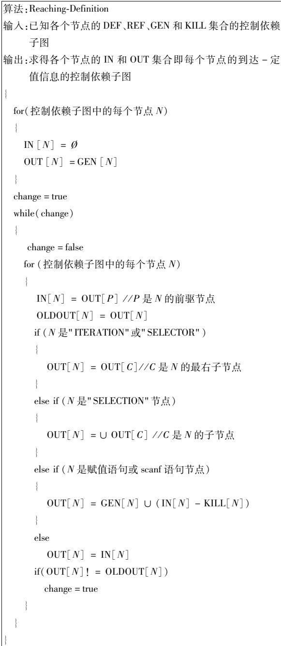
图 5 到达 - 定值信息的求解算法
