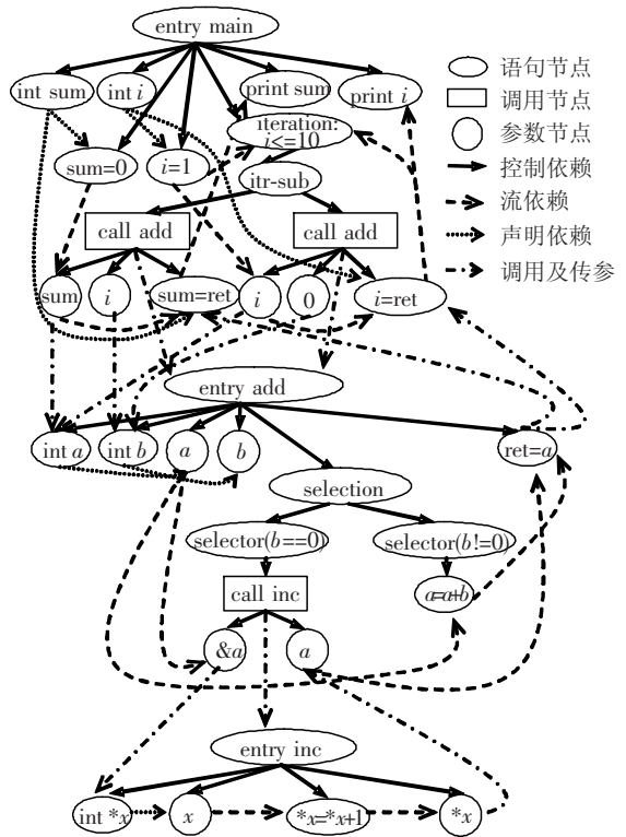
图 9 系统依赖图实例
