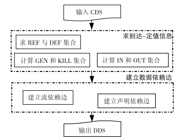
图 3 系统 DDS 构建模型
