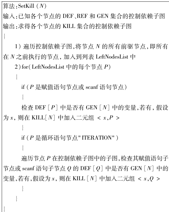
图 4 KILL 集合求解算法
