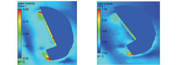
(b) 浮子只有纵摇(左图)和垂荡加纵摇(右图)时的涡量场俯视图
