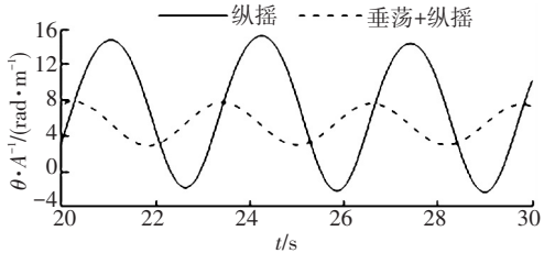
(d) 浮子 3 的纵摇角时历曲线
