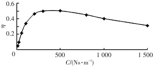
(b) 浮子的垂荡 PTO 阻尼系数-俘获宽度比曲线
