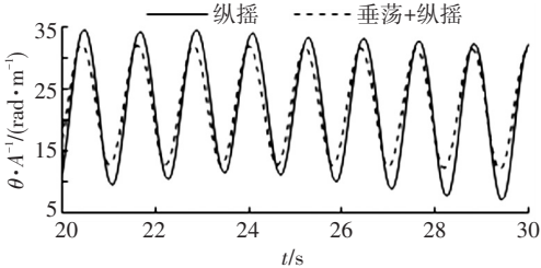
(b) 浮子 1 的纵摇角时历曲线
