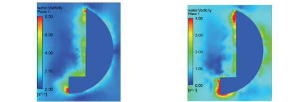
(b) 浮子只有垂荡(左图)和垂荡加纵摇(右图)时的涡量场俯视图
