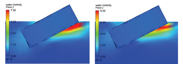
(a) 浮子只有纵摇(左图)和垂荡加纵摇(右图)时的涡量场正视图
