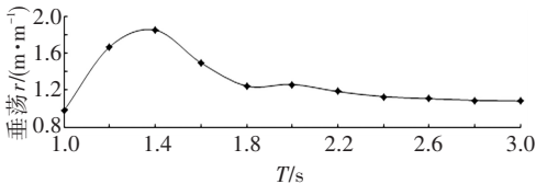
图 4 浮子的垂荡 RAO 曲线
