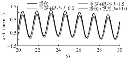
(a) 不同浮子的垂荡位移时历曲线
